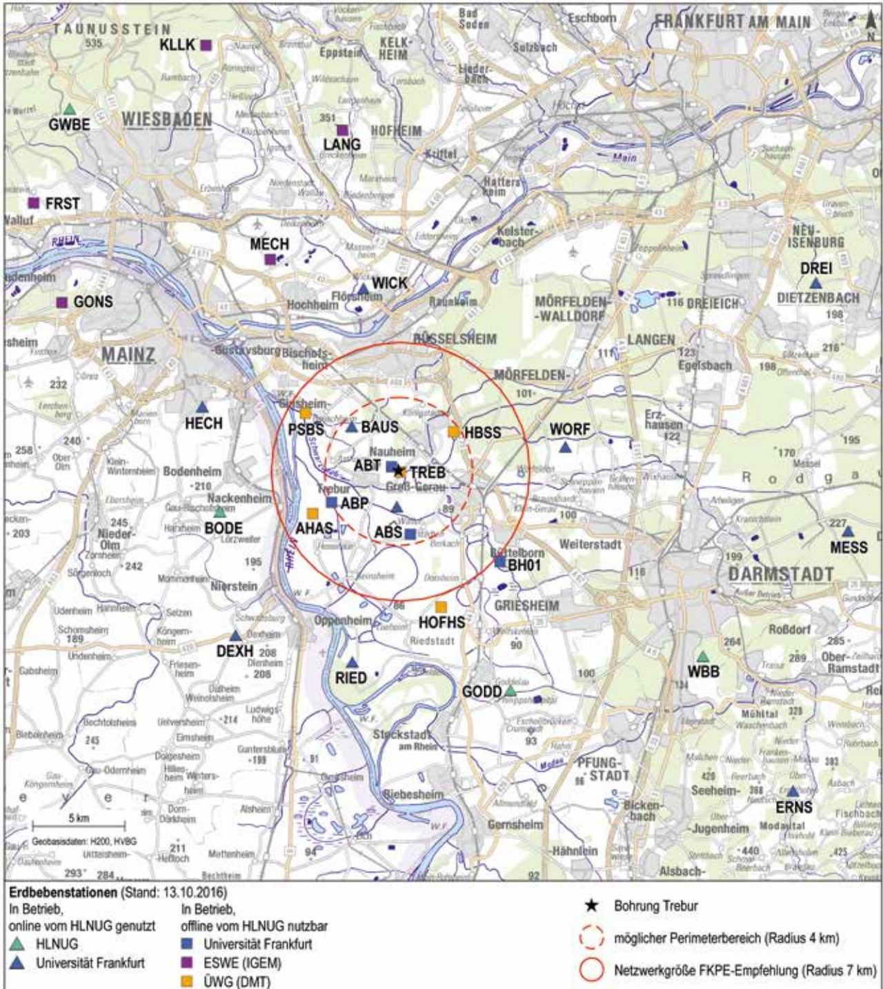
Abb. 3: Netz der beteiligten Messstationen im Untersuchungsgebiet zur Registrierung der natürlichen Seismizität im Verbundprojekt SiMon+.
