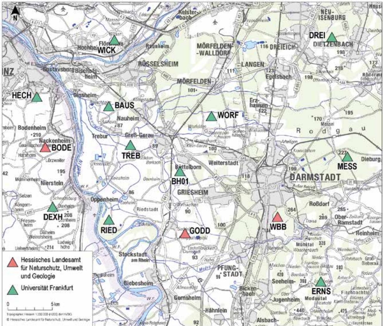
Abb. 4: Karte von der SiMoN+-Webseite: Die beteiligten Messstationen im Untersuchungsgebiet können einzeln aufgerufen werden, um den aktuellen 24-Stundenplot darzustellen.
