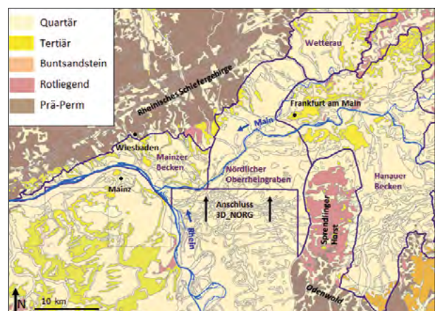
Abb. 1: Übersicht der strukturräumlichen Untergliederung des Senkungsgebietes der Untermainebene (violette Linie). Quelle Strukturraumgrenzen und geologische Karte: Geologische Übersichtskarte des Landes Hessen 1 : 300 000, HLNUG, 2007
