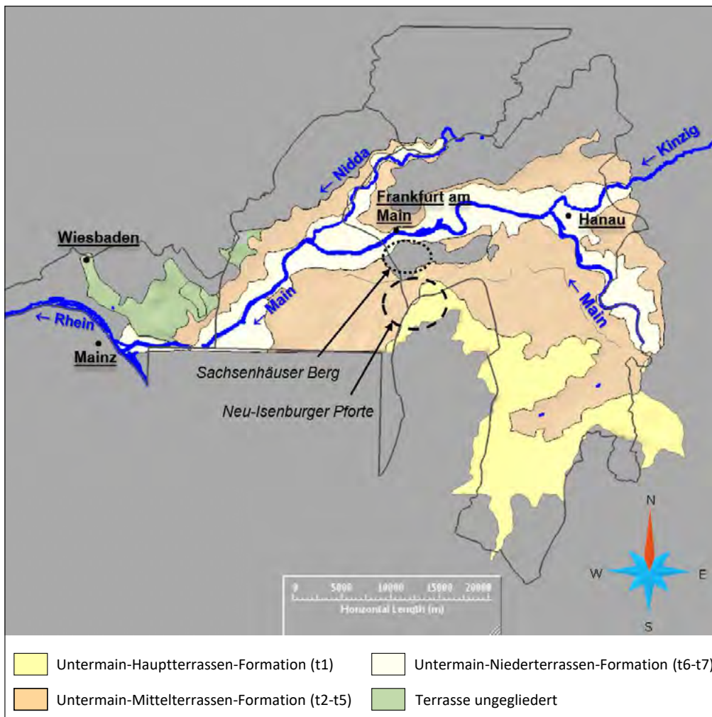
Abb. 4: Basisflächen der Terrassen-Formationen in GOCAD. Quelle Strukturraumgrenzen und geologische Karte: Geologische Übersichtskarte des Landes Hessen 1 : 300 000, HLNUG, 2007
