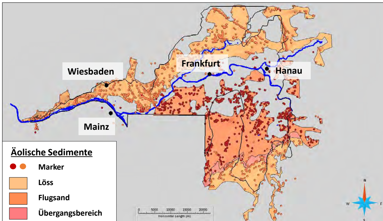
Abb. 5: Modellierte Basisflächen der Löss- und Flugsandverbreitung. Die Punkte geben das Auftreten der Einheiten in den Bohrungen an. Quelle Strukturraumgrenzen und geologische Karte: Geologische Übersichtskarte des Landes Hessen 1 : 300 000, HLNUG, 2007
