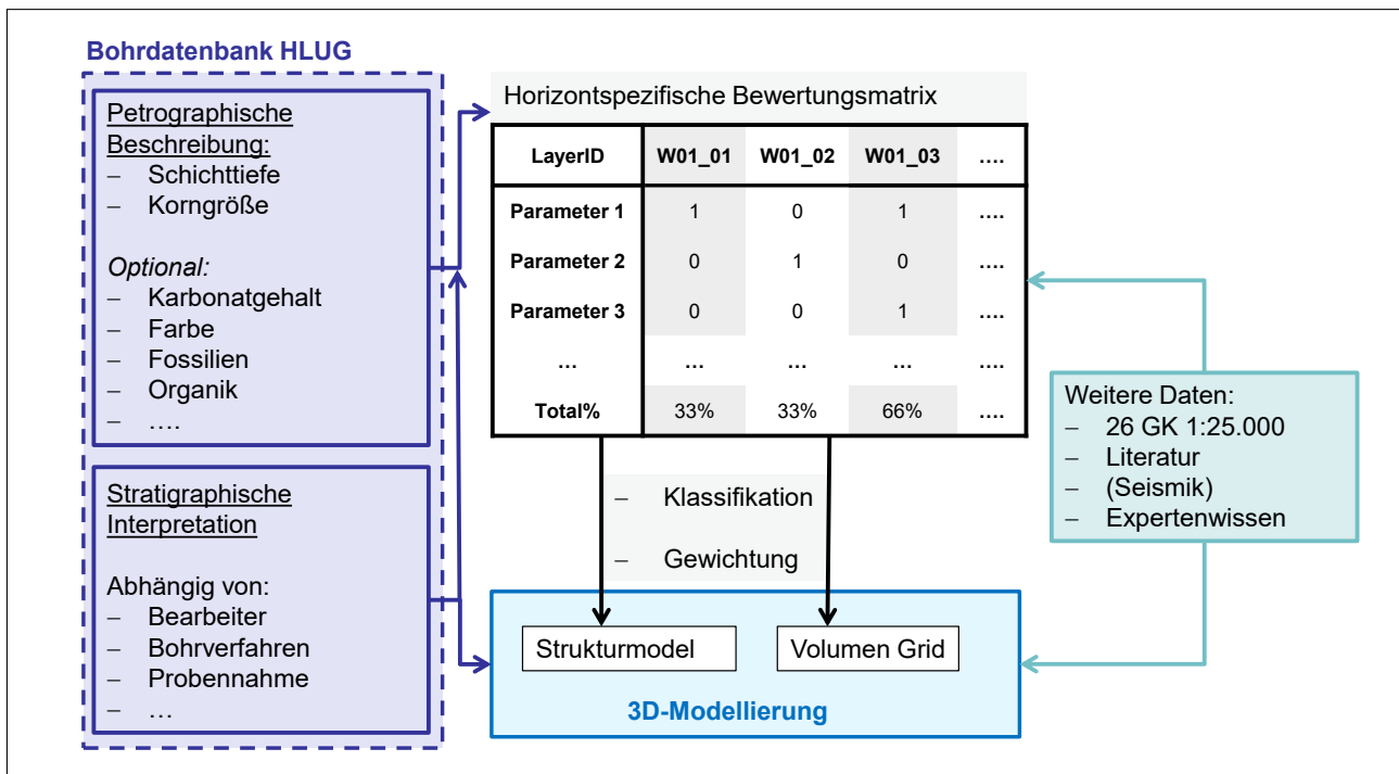
Abb. 2: Schematisches Vorgehen zur Auswahl und Klassifikation der Marker mittels Bewertungsmatrix
