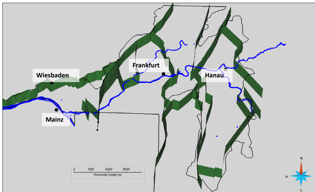
Abb. 7: Modellierte Störungsflächen in GOCAD. Quelle Strukturraumgrenzen und geologische Karte: Geologische Übersichtskarte des Landes Hessen 1:300 000, HLNUG, 2007
