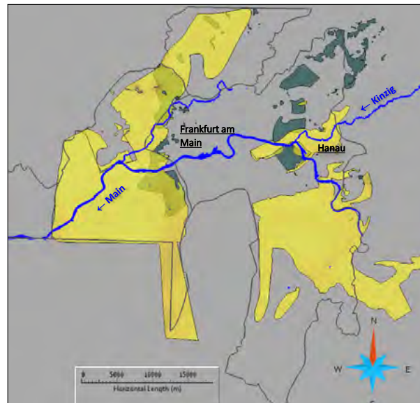
Abb. 6: Verbreitung des Pliozäns (gelb) und des Untermain-Basalts (olivgrün). Vorkommen der Untermain-Basalte im Liegenden des Pliozäns (hellgrün). Quelle Strukturraumgrenzen und geologische Karte: Geologische Übersichtskarte des Landes Hessen 1:300 000, HLNUG, 2007
