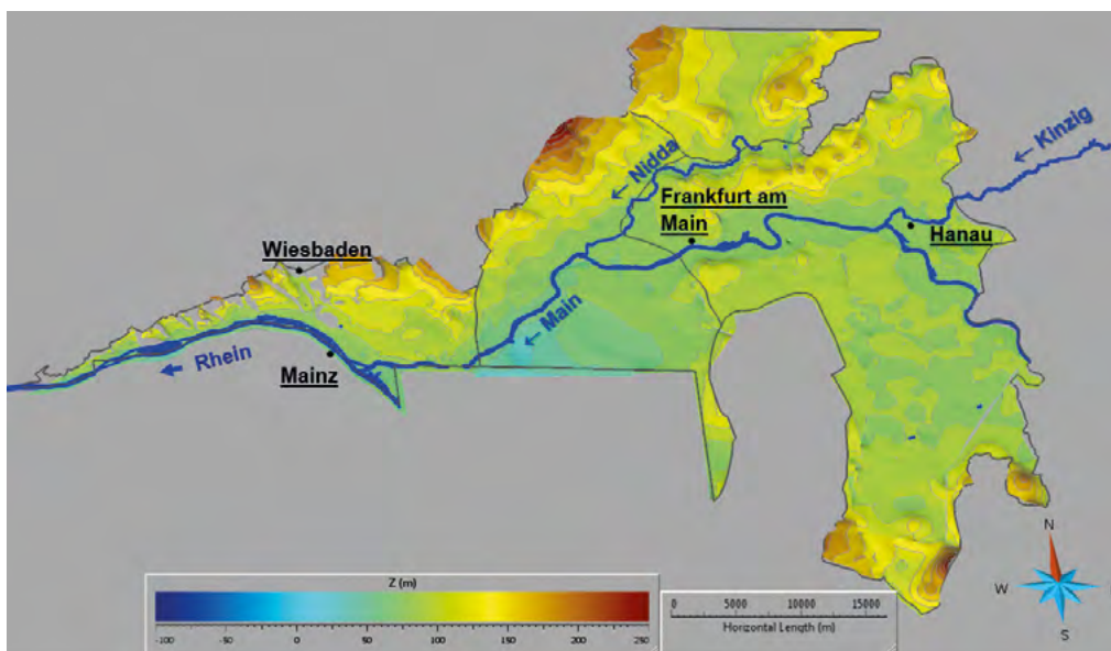
Abb. 3: Basisflächen der quartären Sedimente in GOCAD. Die Farbskala zeigt Tiefenangaben in [m NN]. Quelle Strukturraumgrenzen und geologische Karte: Geologische Übersichtskarte des Landes Hessen 1:300000, HLNUG, 2007
