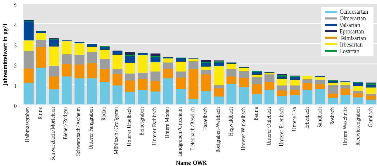
Abb. 4: Sartane (Antihypertonika) in hessischen Fließgewässern. Dargestellt sind nur Wasserkörper mit Summen der Jahresmittelwerte ab 1 µg/l.
