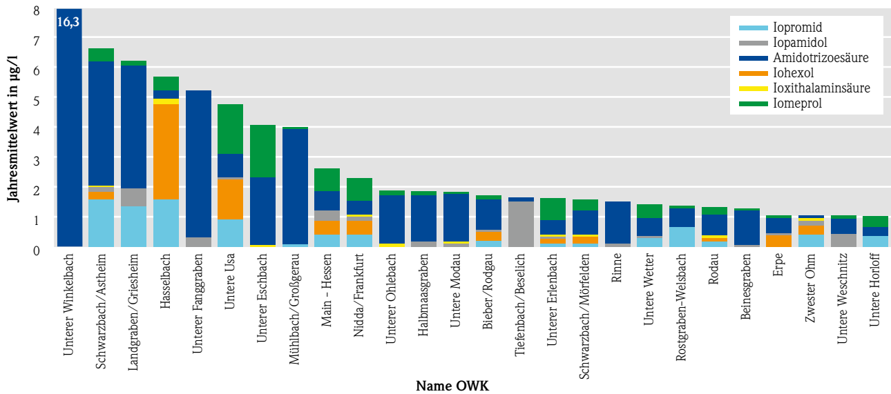
Abb. 3: Röntgenkontrastmittel in hessischen Fließgewässern. Dargestellt sind nur Wasserkörper mit Summen der Jahresmittelwerte ab 1 µg/l.
