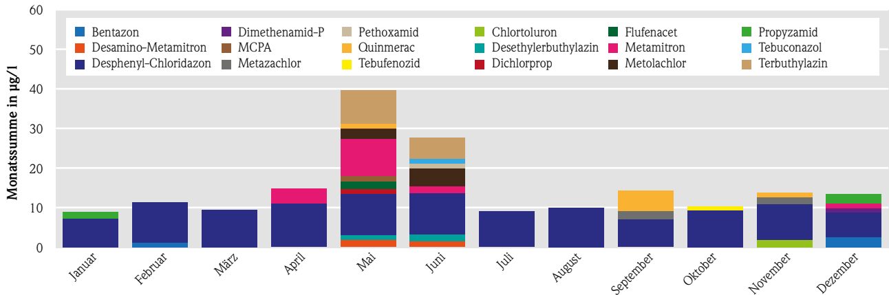
Abb. 2: Monatliche Summen aller PSM-Parameter, die in einem Monat die Top 10 der gemessenen Konzentration erreichen
