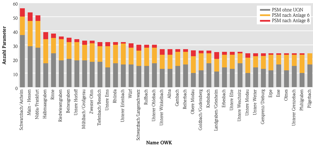
Abb. 1: Anzahl der gefundenen Pflanzenschutzmittel und Metaboliten je Wasserkörper – dargestellt sind hier nur die 36 OWK mit der höchsten Anzahl gefunden PSM
