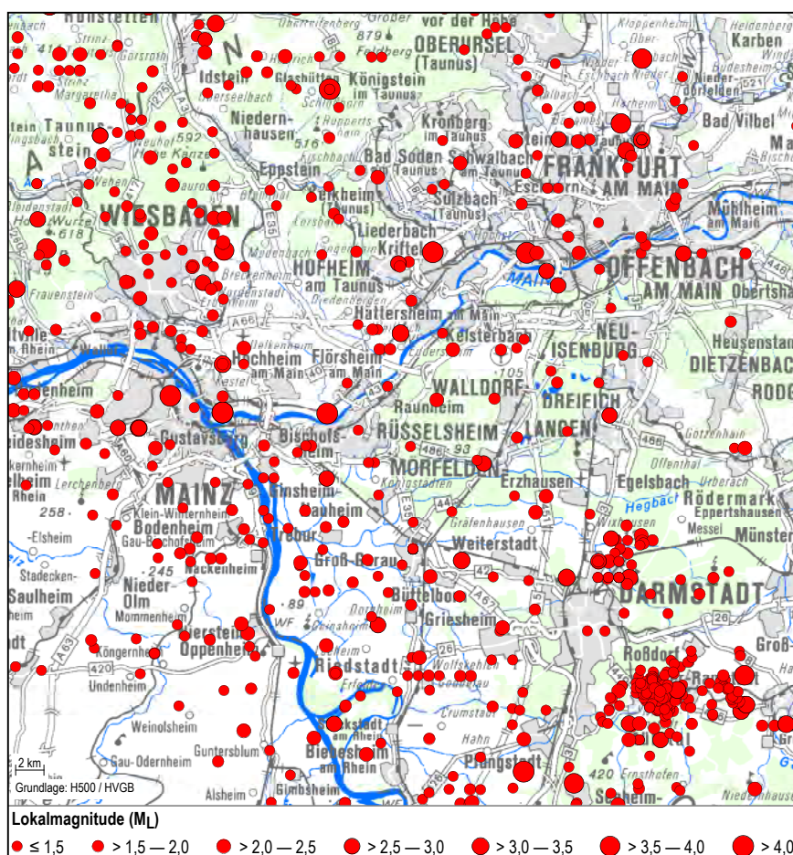
Abb. 6: Erdbebenverteilung von Hessen für die Jahre 858 bis 2017 (Kracht & Homuth 2017)
