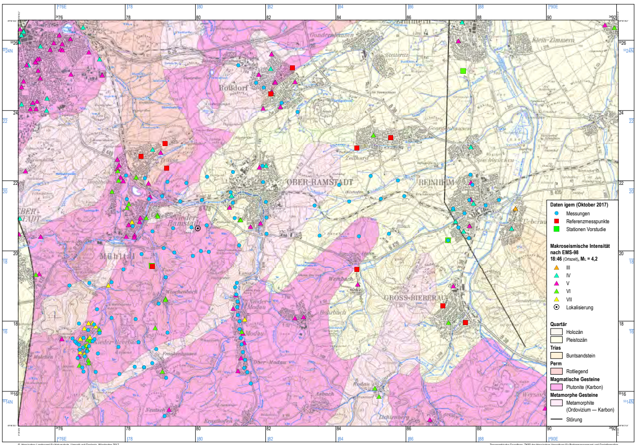
Abb. 8: Geologische Übersichtskarte mit den Untersuchungsgebieten des Projektes SEUSH: „nördlicher Odenwald“ und „Ober-Ramstadt“. Es sind die Positionen der registrierten Schadens- und Intensitätsmeldungen eines lokalen seismischen Ereignisses sowie alle innerhalb des Kartengebiets liegenden Messpunkte aufgeführt.
