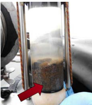
Abb. 4: Beprobung von Main-Sediment mittels Sedi-Corer (Fa. Uwi-tec) © BCE Koblenz
