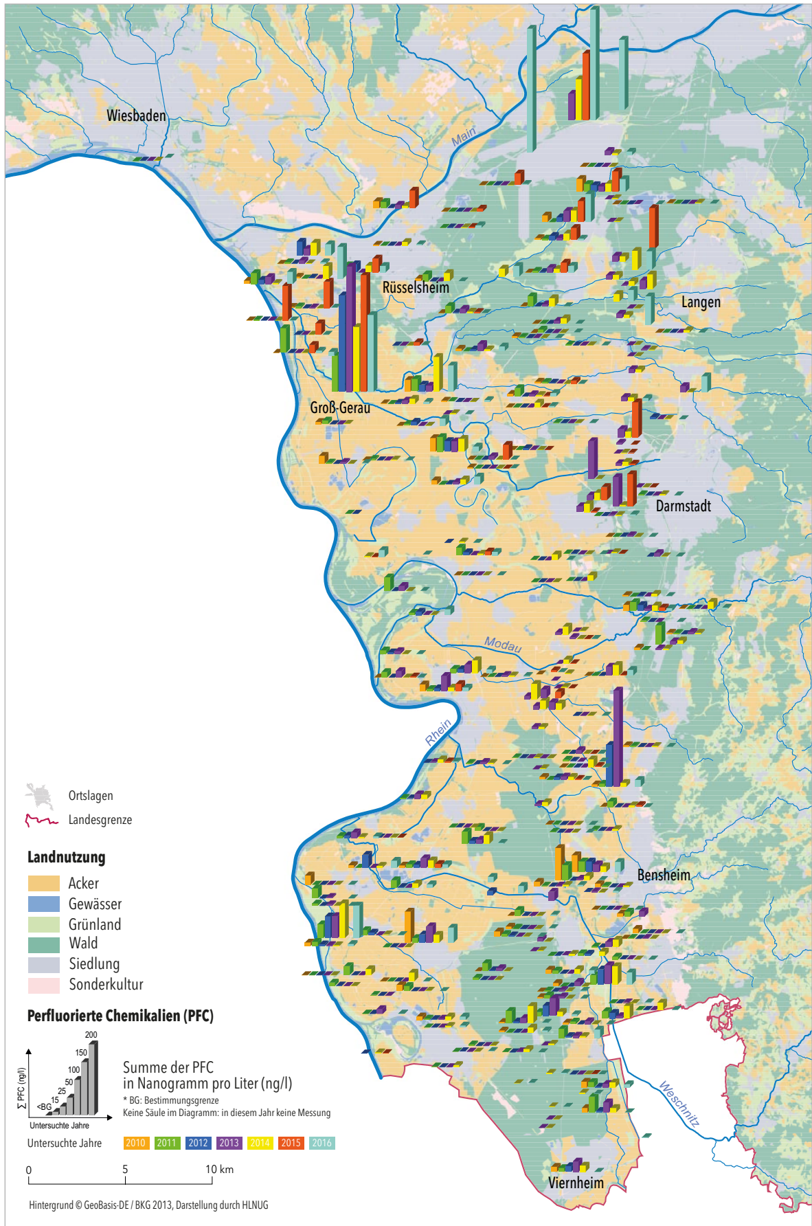
Summe aller PFC-Einzelparameter der Jahre 2010–2016, Detailkarte Hessisches Ried
