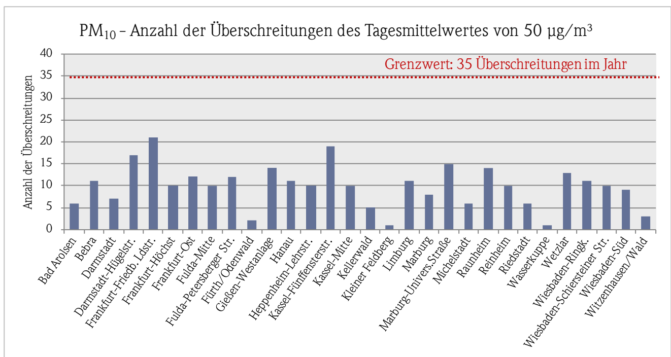
Abb. 6: Feinstaub (PM 10 ) – Überschreitungen des Grenzwertes für die kurzfristige Belastung im Messjahr 2013
