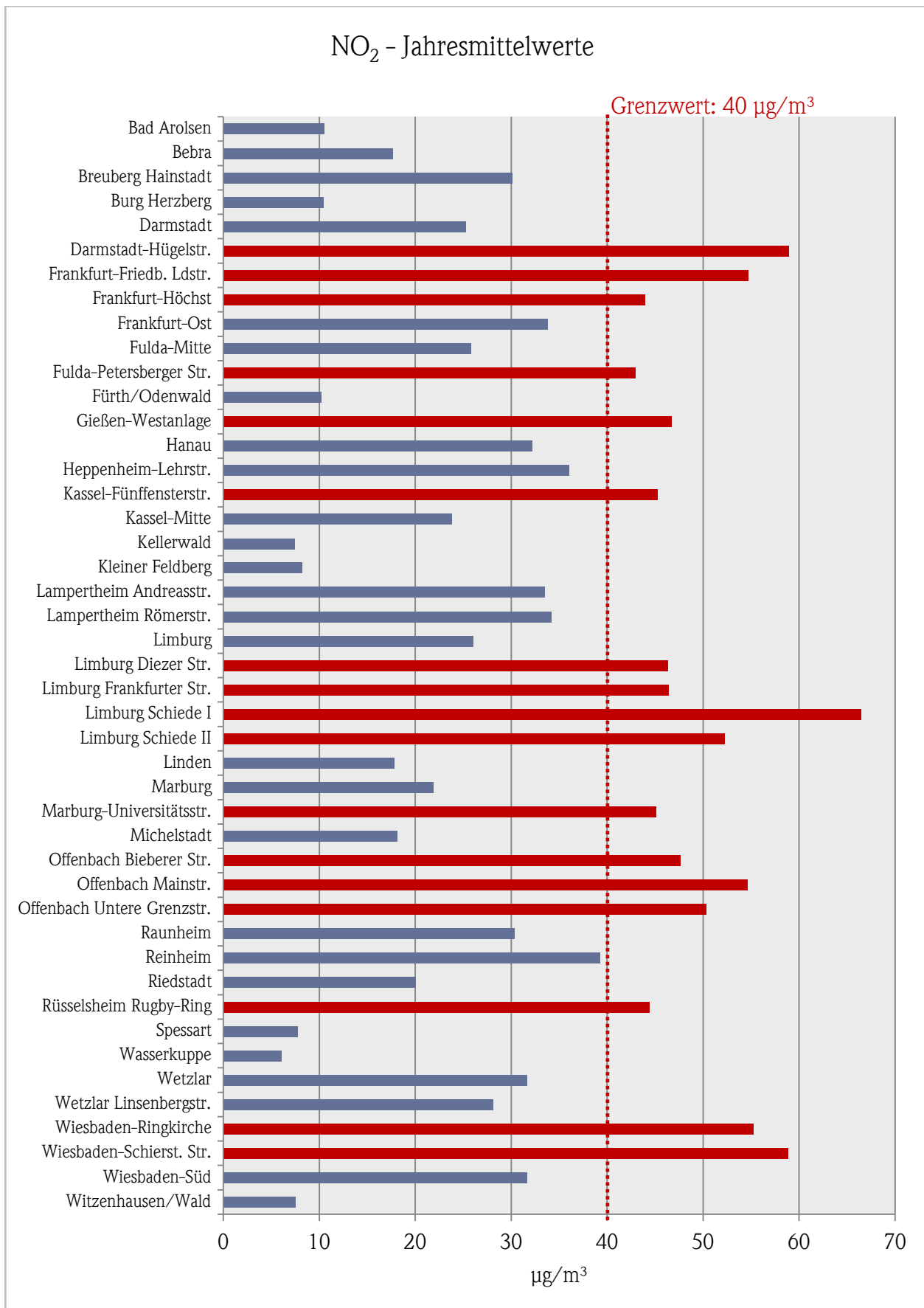
Abb. 7: Stickstoffdioxid (NO 2 ) – Überschreitungen des Grenzwertes für die langfristige Belastung im Messjahr 2013
