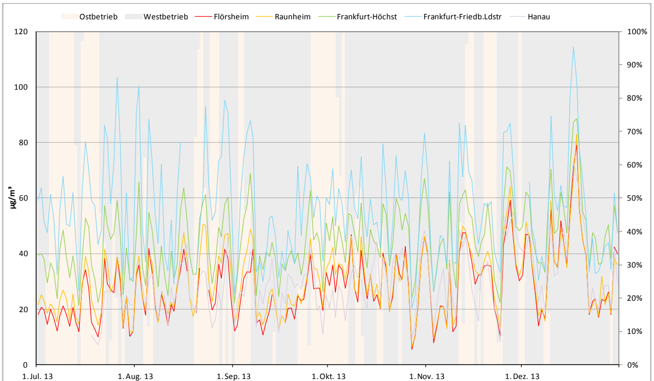
Abb. 8: Zeitlicher Verlauf der NO 2 -Tagesmittelwerte sowie die Verteilung der beiden möglichen Betriebsrichtungen bei Anflug auf den Flughafen Rhein-Main in Prozent, Station Flörsheim im Vergleich zu umliegenden Stationen
