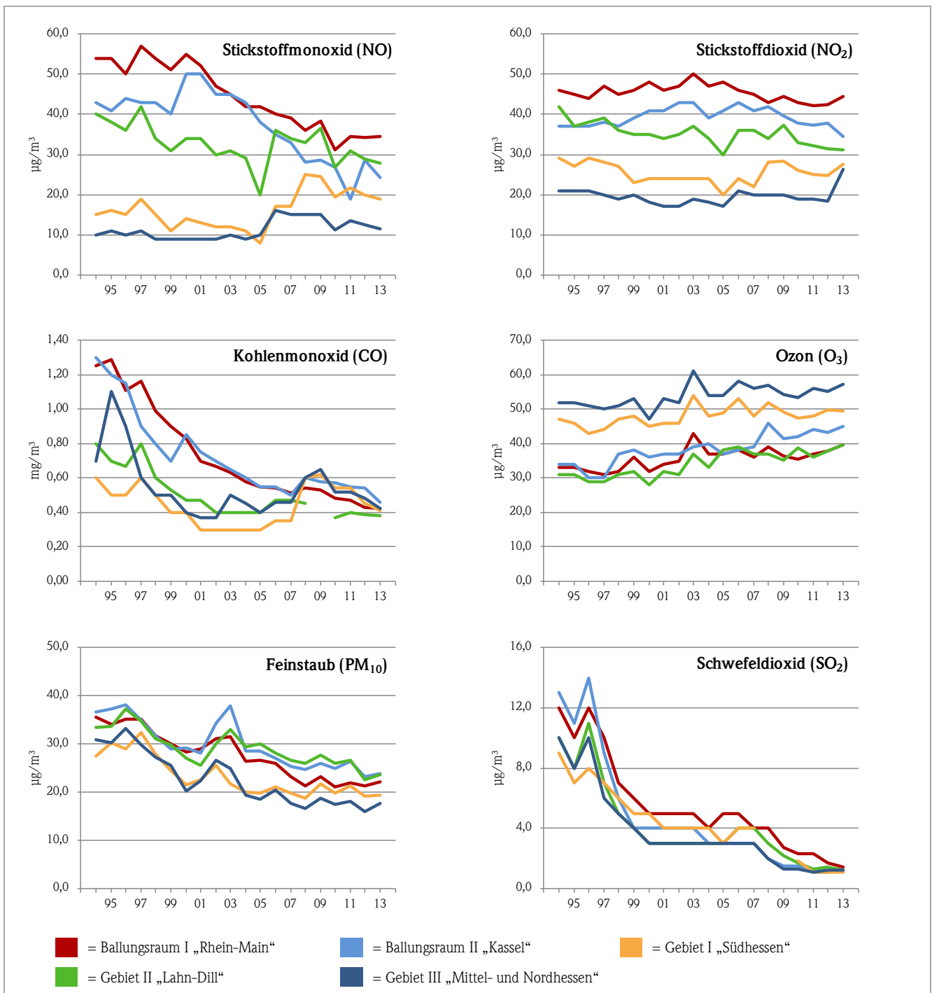
Abb. 5: Zeitreihen der Jahresmittelwerte 1994–2013
