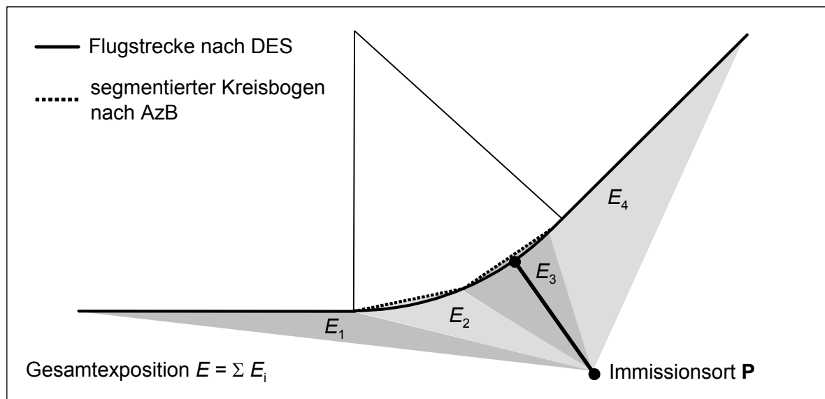
Abbildung 1 : Prinzip der Segmentierung am Beispiel der Zerlegung eines kreisbogenförmigen Flugstreckensegments in zwei lineare Teilsegmente
