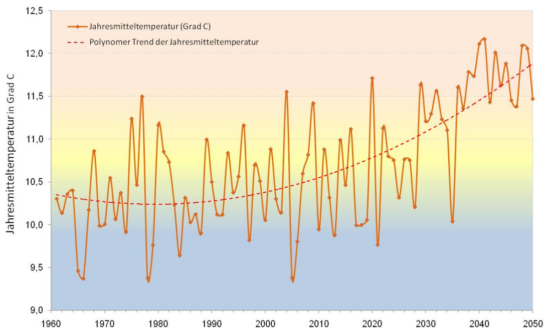
Abb. 4: Modellierte Jahresmitteltemperatur der Klimastation Mannheim (Szenario A1B)
