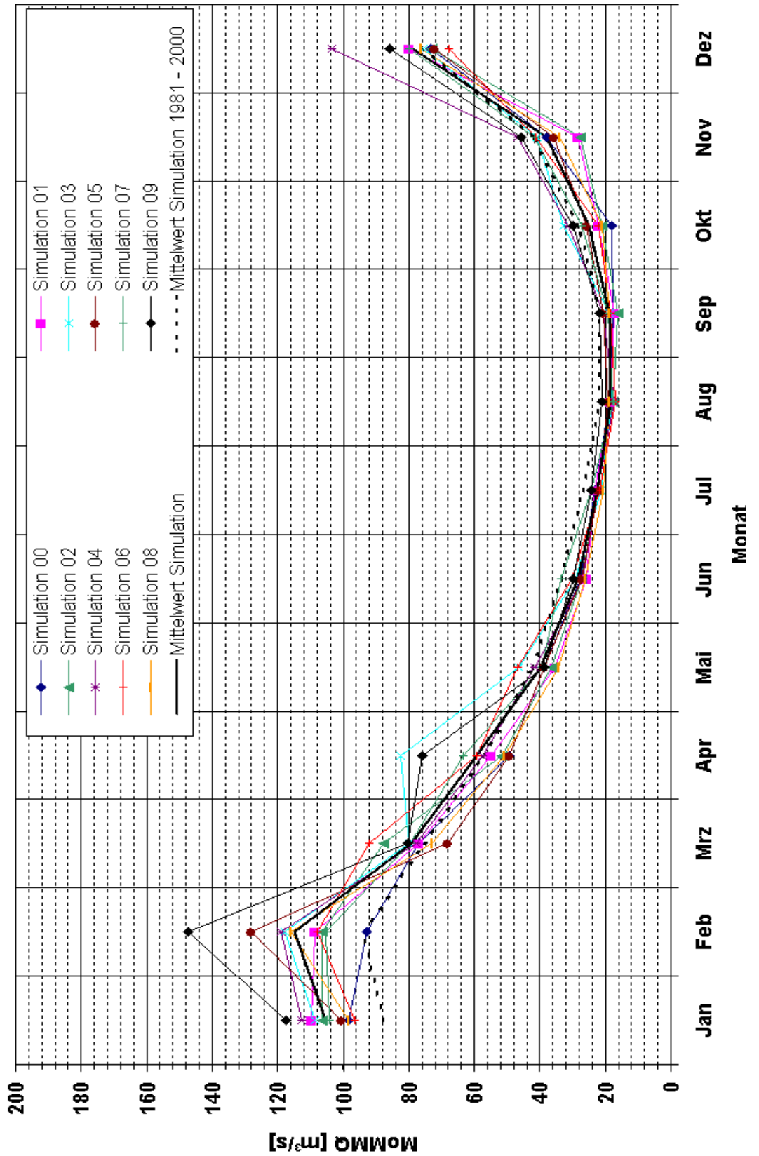
Mittlere monatliche Mittelwasserabflüsse 2011 - 2020 MoMMQ Pegel Kalkofen, Lahn Eingangsdaten nach Enke 2004 (Meteo-Research)
