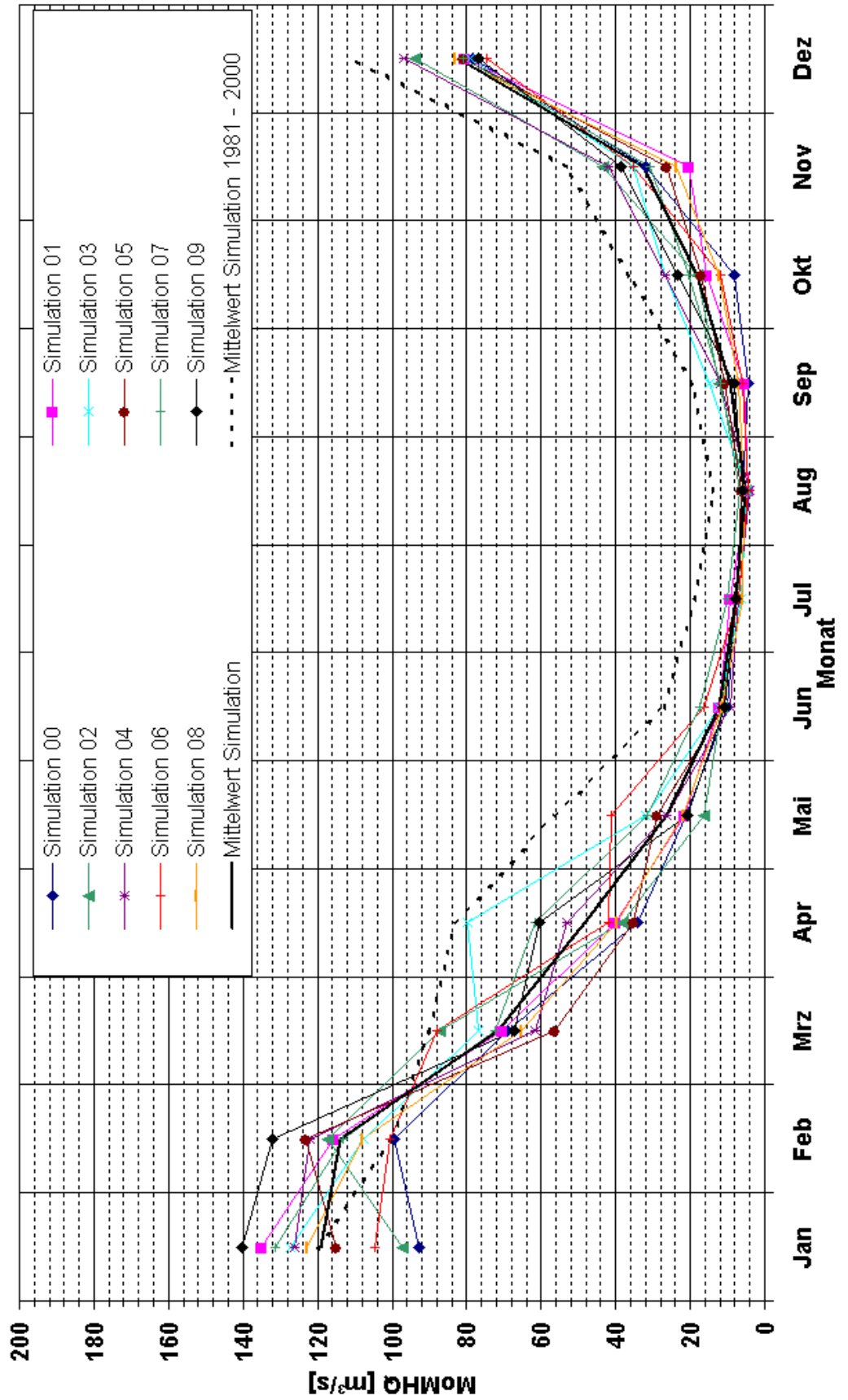
Mittlere monatliche Hochwasserabflüsse 2011 - 2020 MoMHQ Pegel Schmittlotheim, Eder Eingangsdaten nach Enke 2004 (Meteo-Research)
