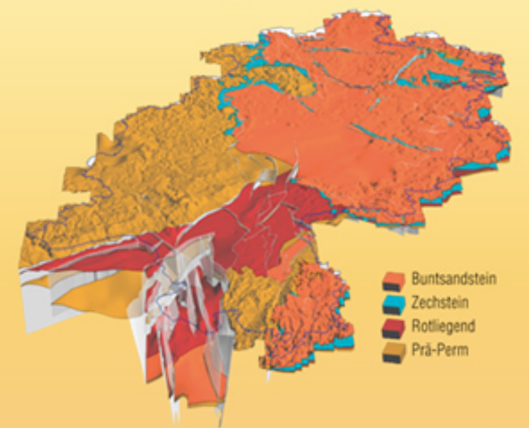
Blick Richtung Norden auf Modellschichten des geologischen 3-D-Modells (dreifach überhöht), grau: Störungsflächen (ARNDT 2011)
