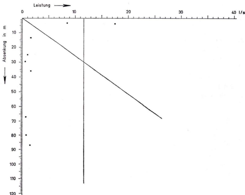
Abb. 8. Leistungsdiagramme von Brunnen im Rheinischen Schiefergebirge (Nordhessen).
