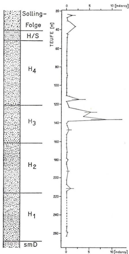
Abb. 4. Durchlässigkeit und petrographische Ausbildung der Solling- und Hardegsen-Folge in Bg. Beberbeck.
