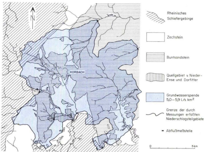
Fig. 2. Grundwasserspender im Gebiet von Korbach
