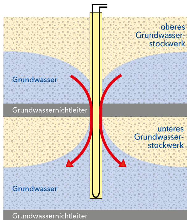
Abb. 8: Unzureichend abdichtete Erdwärmebohrung. Grundwasser strömt in diesem Beispiel von einem höheren in ein tieferes Grundwasserstockwerk. Bei einem höheren Druckniveau im tieferen Stockwerk (gespanntes Grundwasser) kann auch ein Aufstieg des Grundwassers in das obere Stockwerk oder sogar bis zur Geländeoberfläche stattfinden.
