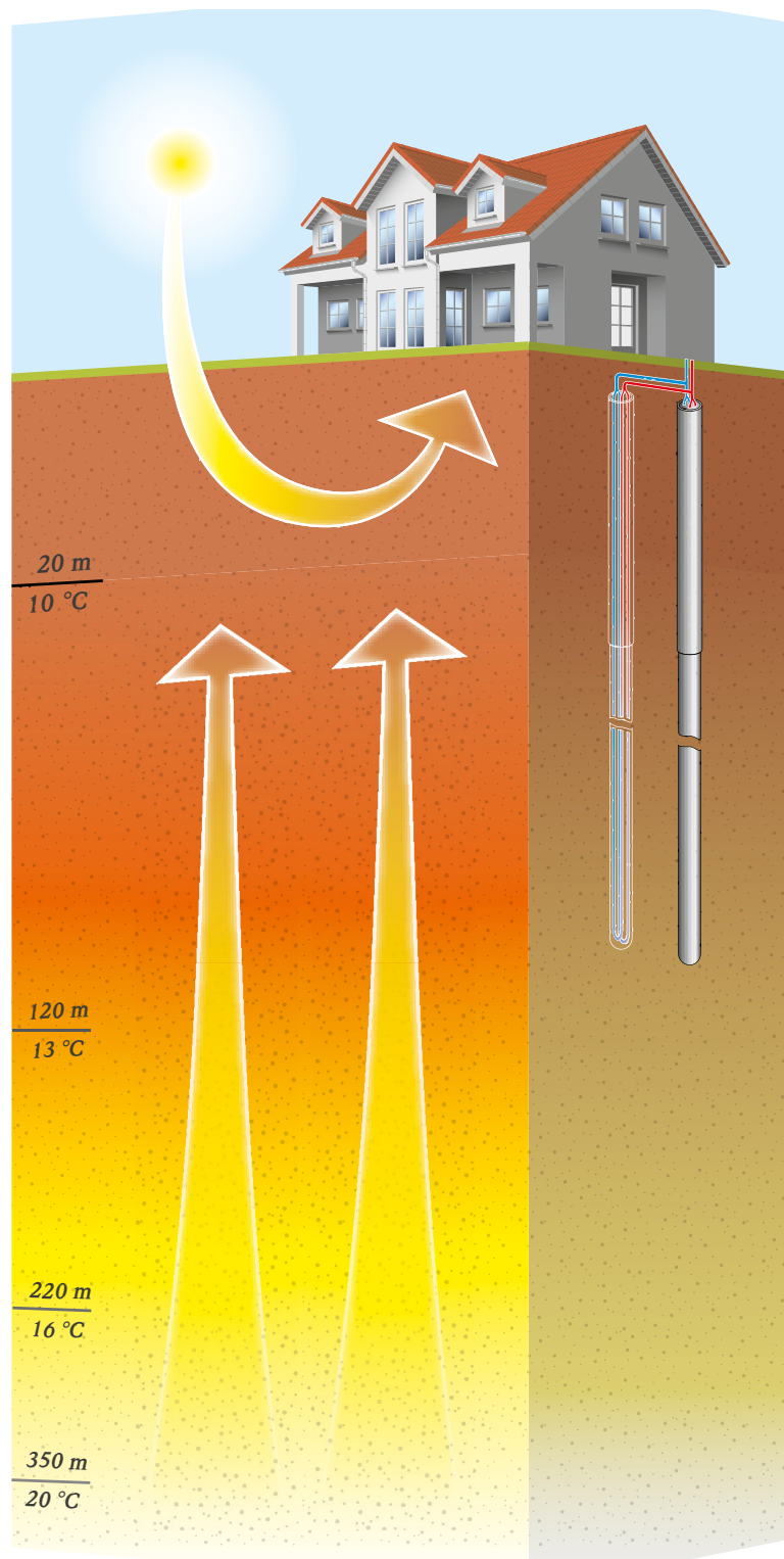
Abb. 1: Einflussbereiche des solaren und terrestrischen Wärmestroms. Im Einflussbereich des terrestrischen Wärmestroms steigt die Temperatur im Schnitt um 3 °C pro 100 m Tiefe. Hier ist die Temperatur keinen jahreszeitlichen Schwankungen unterworfen.
