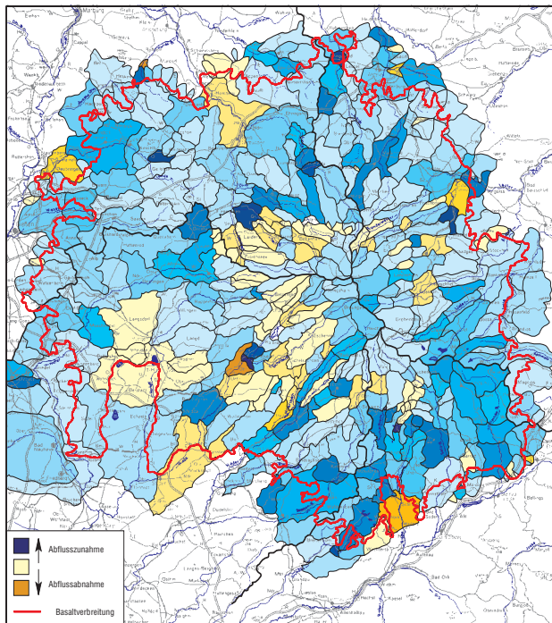
Abflussverluste und Abflusszuwächse bei Fließgewässern bezogen auf oberirdische Einzugsgebiete.
