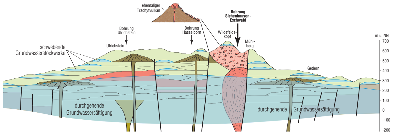
Hydrogeologischer Schnitt durch den Vogelsberg.
