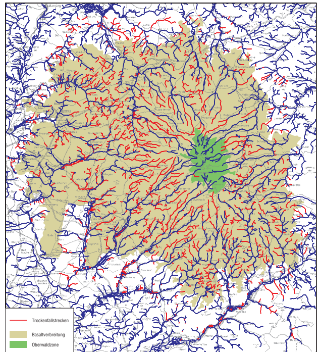
Trockengefallene Fließgewässer im Spätsommer des Jahres 1976.
