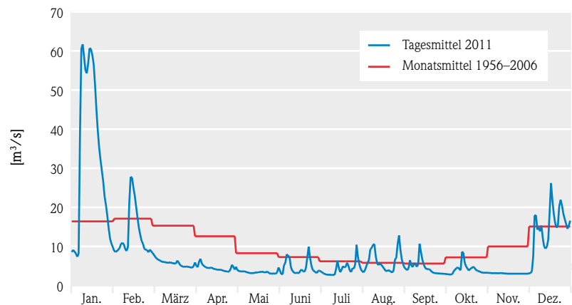
Abb. 4: Abfluss (Tagesmittel 2011 und Monatsmittel 1956–2006) am Pegel Bad Vilbel (Nidda).
